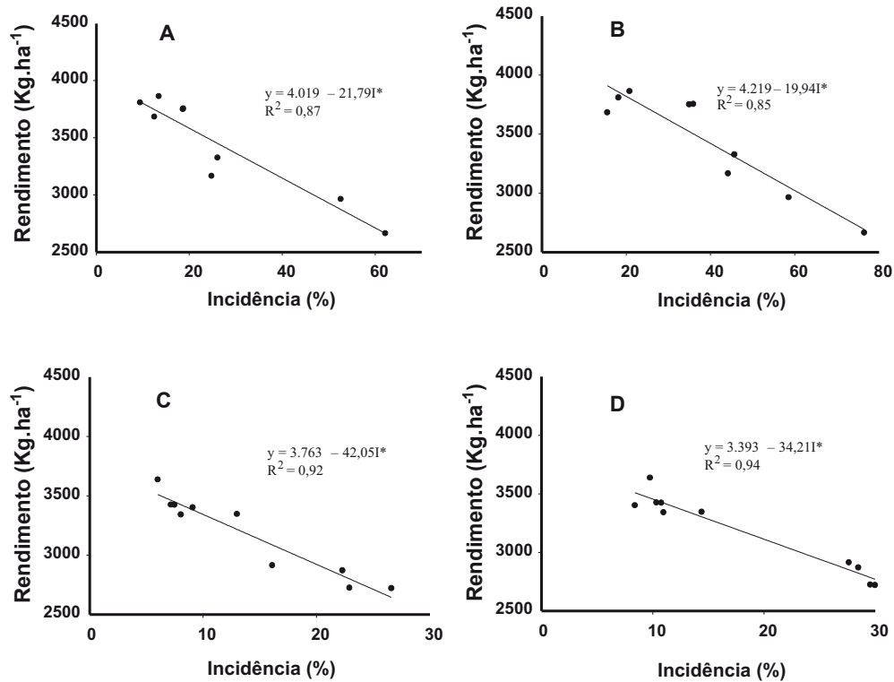
FIG. 1 - Relação entre rendimento de grãos e incidência de doenças fúngicas foliares na cultivar de trigo Ônix nos estádios de um quarto da inflorescência emergida ( A . 2005; C . 2006), emborrachamneto ( B . 2006) e início da antese ( D . 2006) em São José do Cerrito. Lages SC, 2007.
