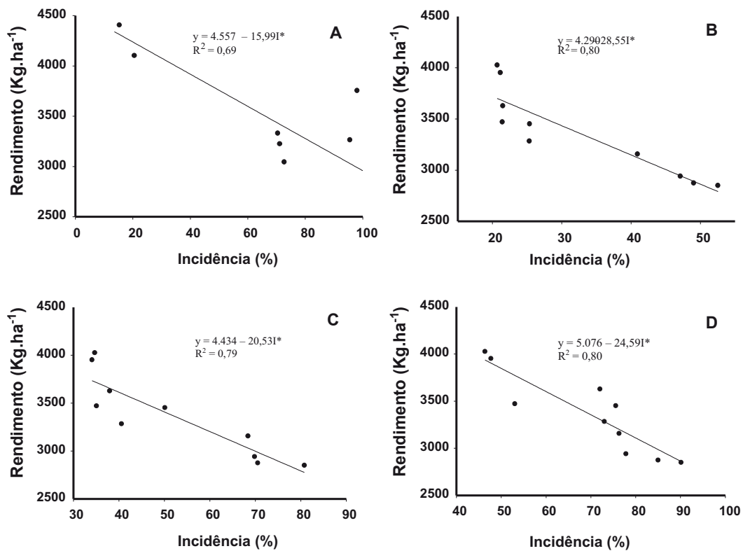
FIG. 2 - Relação entre rendimento de grãos e incidência de doenças fúngicas foliares na cultivar de trigo BRS Louro nos estádios de emborrachamneto ( A . 2005; C . 2006) e um quarto da inflorescência emergida ( B . 2005; D . 2006) em São José do Cerrito. Lages SC, 2007.
