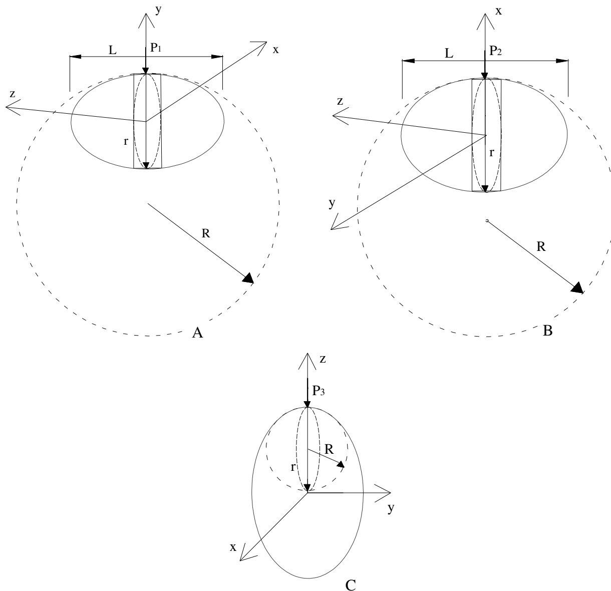
FIGURA 4. Raios de curvatura do grão de soja na região de contato “produto-placa compressora”, usados na determinação dos “módulos proporcionais de deformidade”. (A) compressão na posição P_1 ; (B) compressão na posição P_2 , e (C) compressão na posição P_3 .
