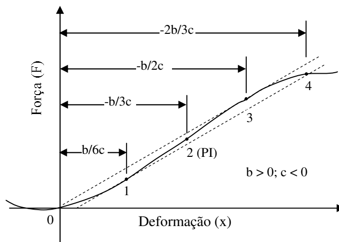
FIGURA 1. Ilustração da curva força vs deformação do modelo F = ax + bx^2 + cx^3 ; para b > 0 e c < 0 ; primeira região inclui a curva da origem até o ponto 1; segunda região inclui a curva dos pontos 1 a 3; terceira região inclui o ponto 3 até o final do teste; PI = ponto de inflexão (HENRY et al., 1996).
