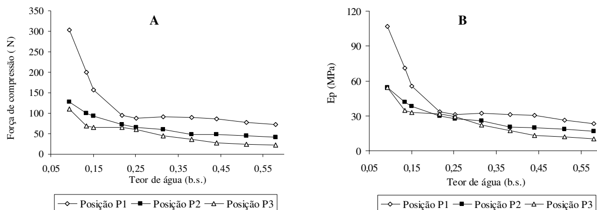
FIGURA 5. Valores médios da força máxima de compressão (A) e do módulo proporcional de elasticidade - E_p (B) de grãos de soja em função do teor de água para diferentes posições de compressão.
