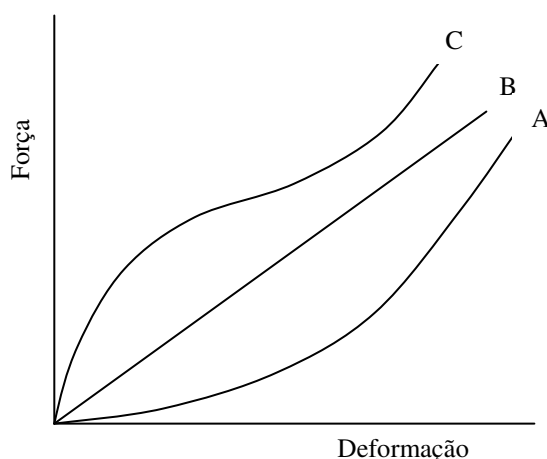
FIGURA 2. Três curvas típicas do comportamento força-deformação para alimentos (BOURNE, 2002).
